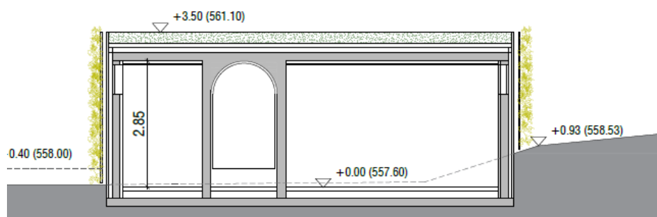
SCHNITT | SEZIONE A-A
