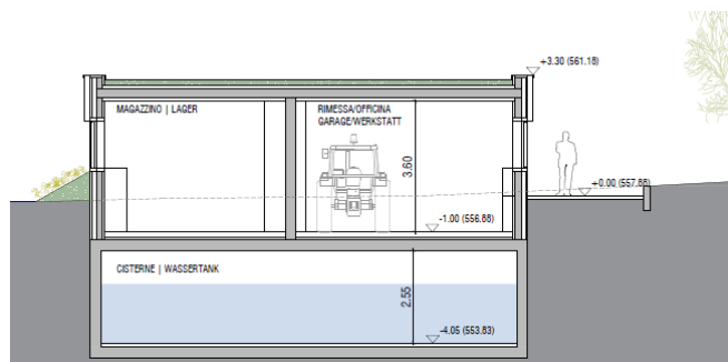
SCHNITT | SEZIONE C-C
