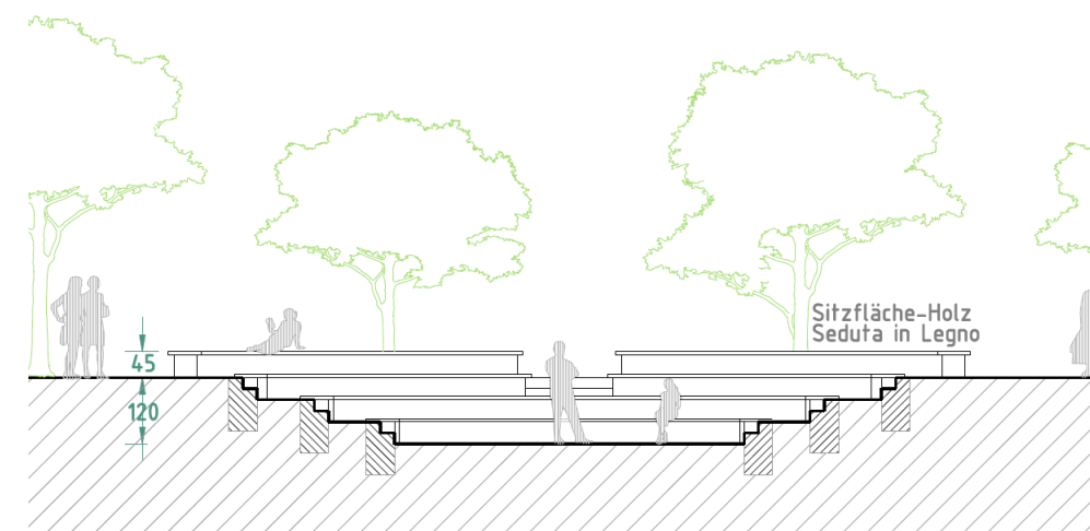
SCHNITT/SEZIONE
