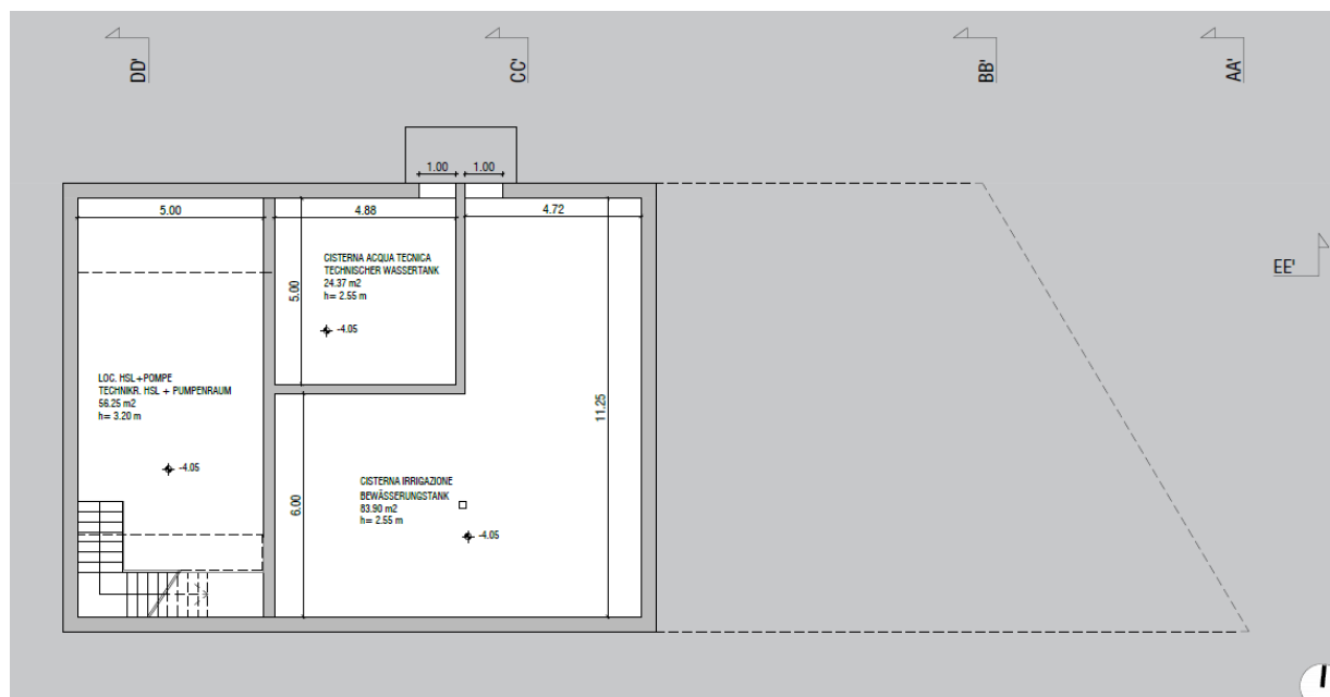
UNTERGESCHOSS | PIANO INTERRATO
