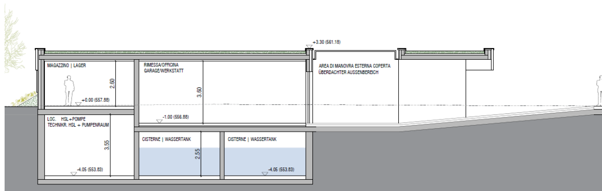
SCHNITT | SEZIONE E-E
