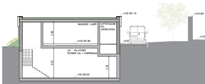
SCHNITT | SEZIONE D-D
