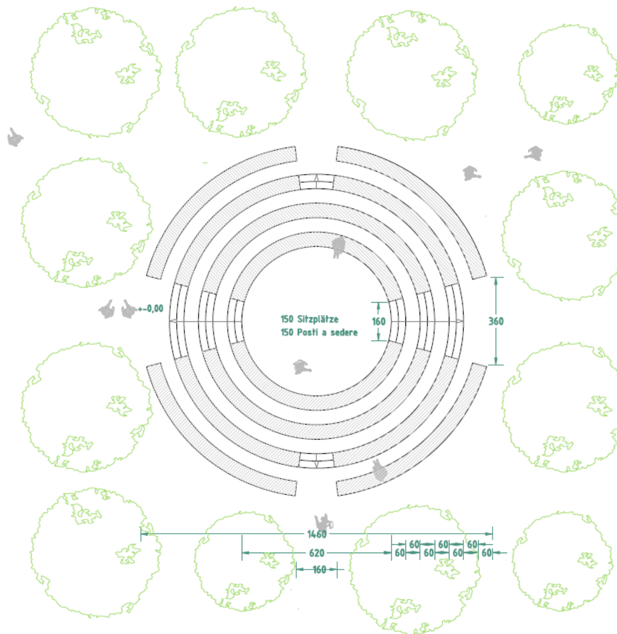
GRUNDRISSE/PIANTA
