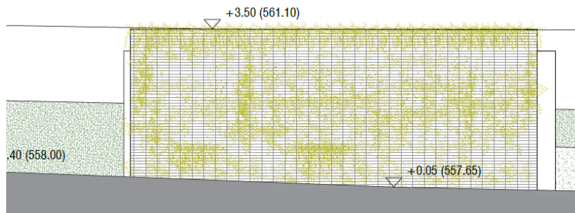
ANSICHT WEST | PROSPETTO OVEST
