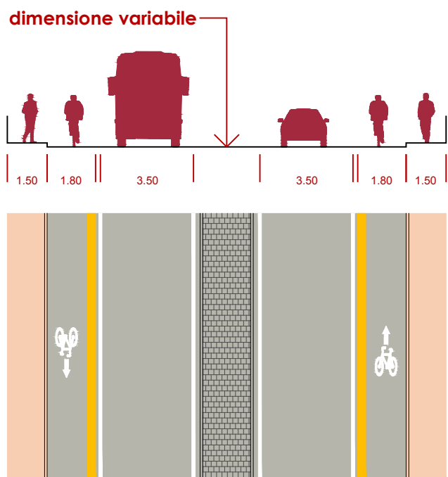
sezione via Brennero | ipotesi A tra via Gasser e via Lechner
