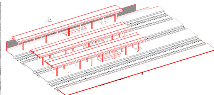
Spaccato Assonometrico
